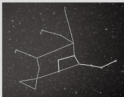
おおぐま座
