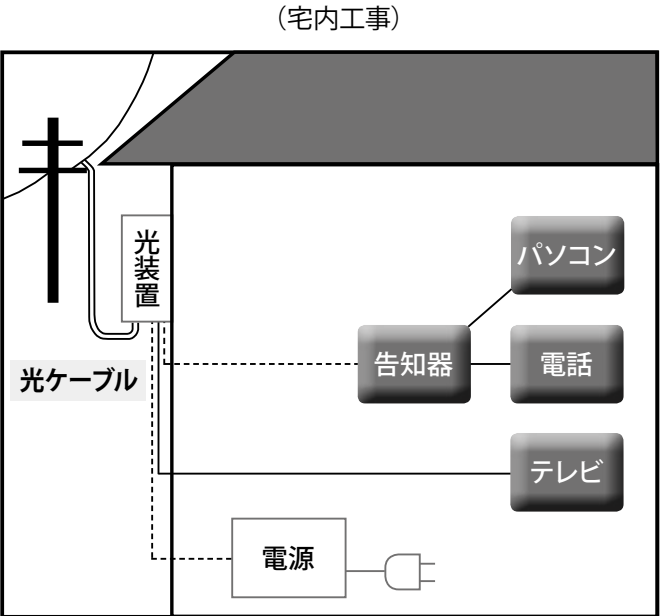
▲光装置・LAN ケーブル・電源などを設置
